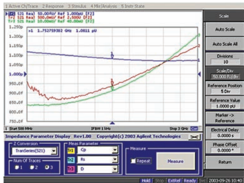
阻抗值显示
