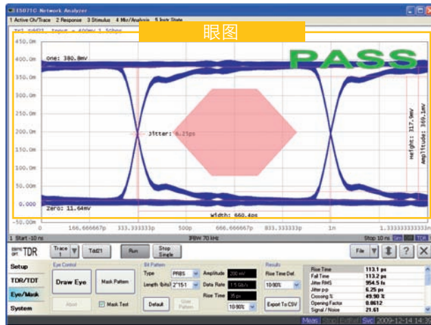
可使用虚拟比特码型发生器进行仿真眼图分析
