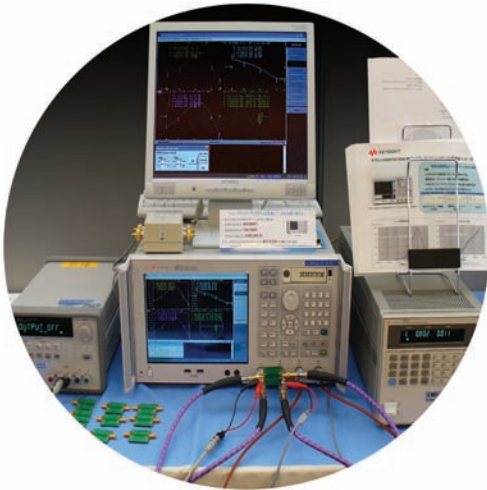
直流偏置的测量设置
