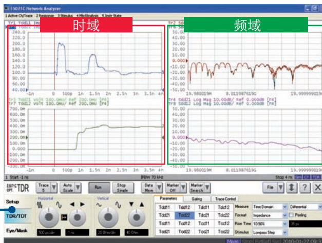
可同时进行时域分析和频域分析
