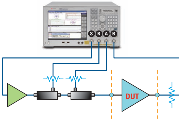
使用外部测试仪模式进行大功率测量
