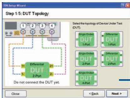
“设置向导”可引导用户完成所有必需的步骤。
