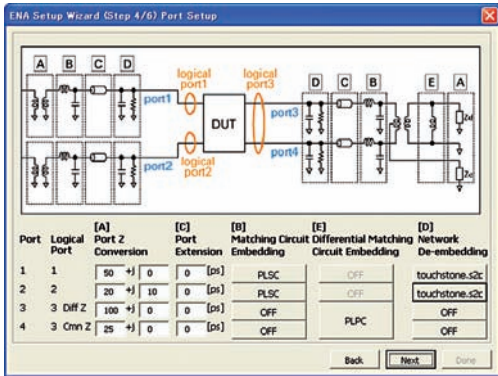
使用设置向导软件进行夹具仿真器的设置
