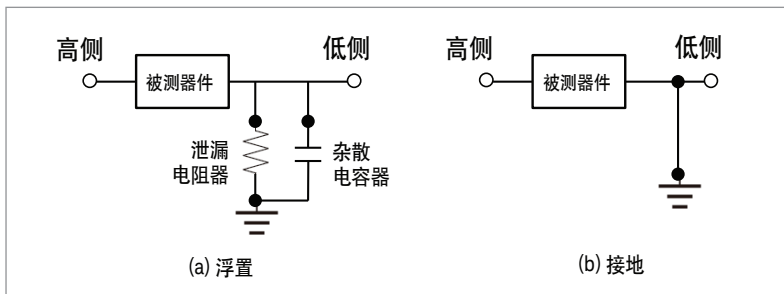
图 2. 浮置和接地测量示例。
