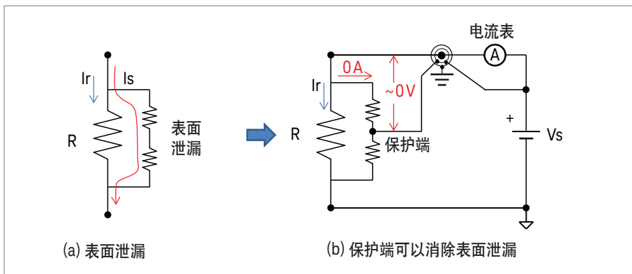
图 7. 高电阻器件等效电路示例。
