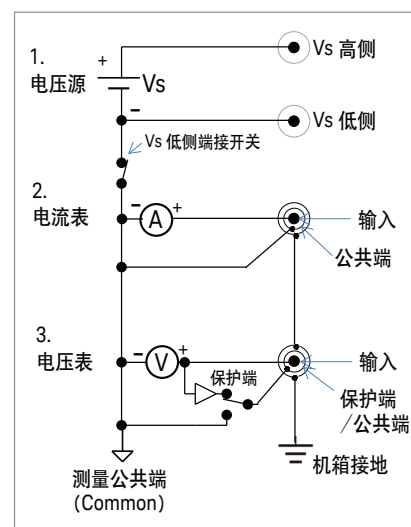
图1. B2985A/87A测量资源。
