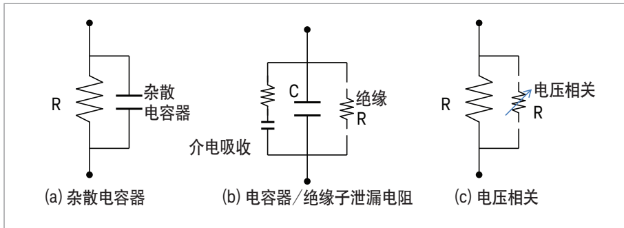
图 5. 在测量高电阻器件时遇到的寄生元件的示例。
