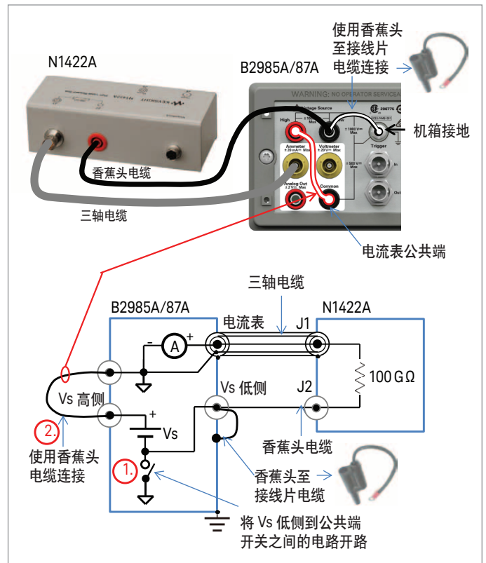
图9. 高电阻测量装置 (接地)。
