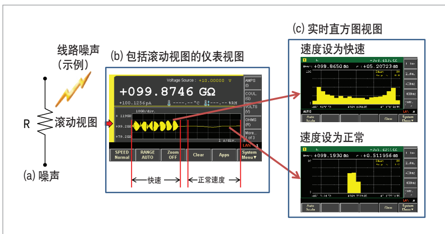
图 4. View (视图) 功能使噪声源分析变得轻而易举。
