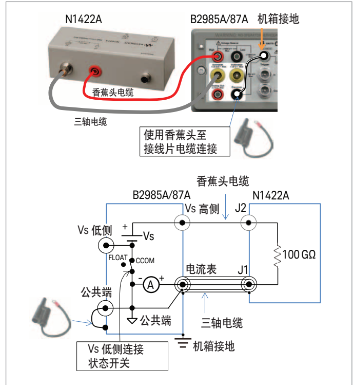
图 8. 高电阻测量的线缆连接和测试资源图(浮置)。
