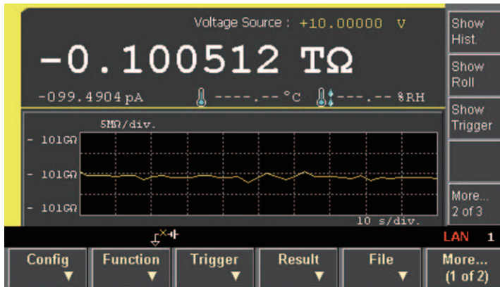
图 11. 接地高电阻测试示例。
