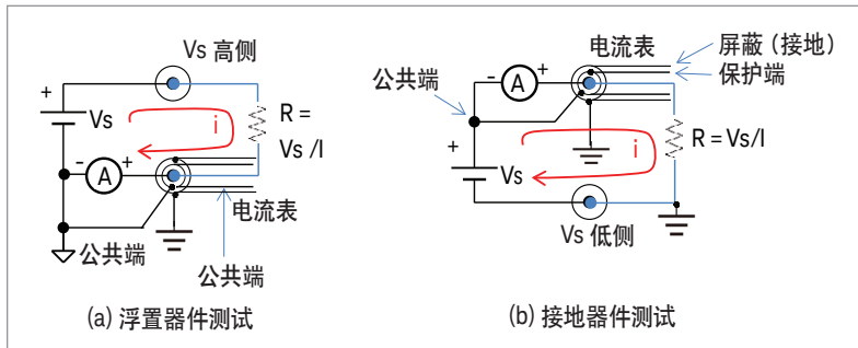
图 3. 高电阻测量模式。
